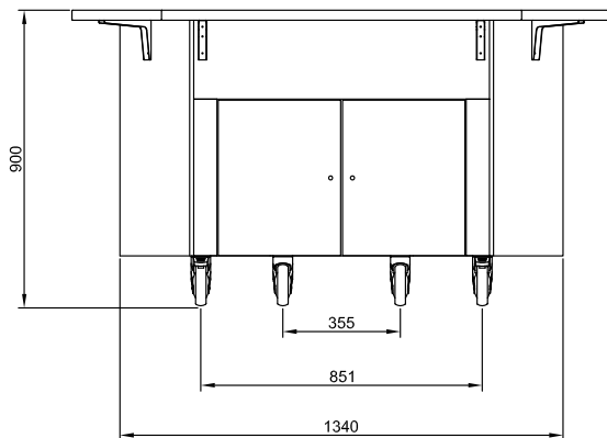
Zij aanzicht
